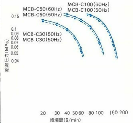
給湯ポンプ性能曲線
